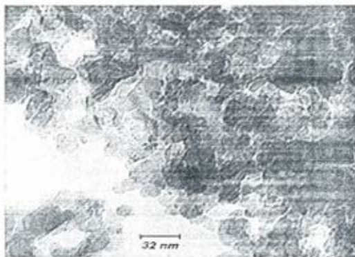
شکل ۱- تصویر میکروسکوپ الکترونی عبوری از نانوذرات آلومینا
