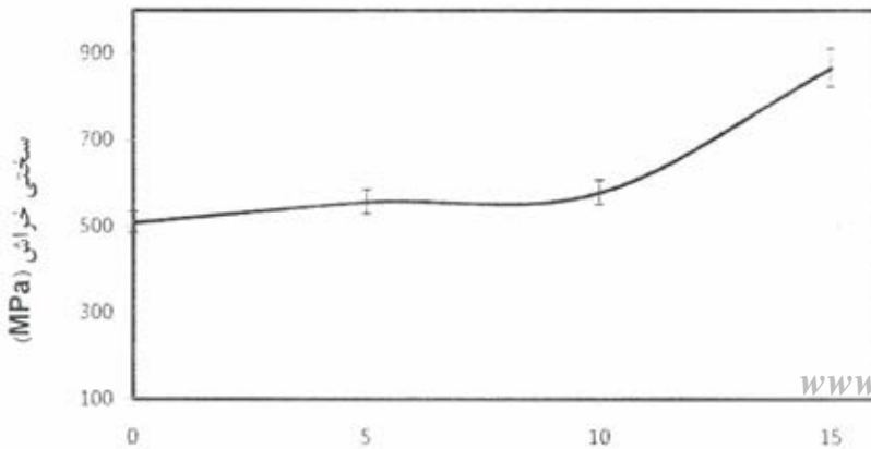
شکل ۵- نمودار سختی خراش بر حسب درصد وزنی نانوذرات آلومینا.
